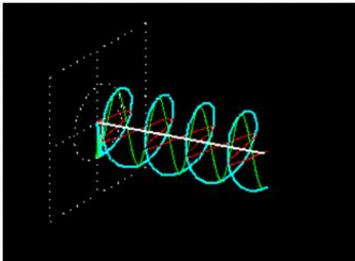
Polarisation Circulaire Gauche LHCP sur deux antennes antagonistes La polarisation tourne dans le sens inverse des aiguilles d'une montre face au réflecteur & collecteur des ondes
